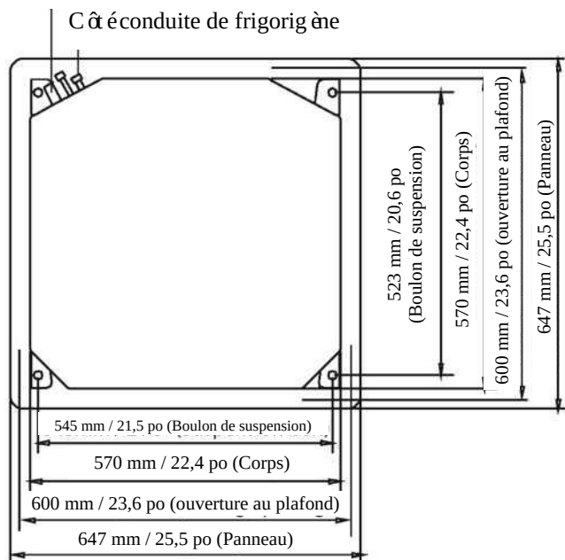
Modèles Compacts dimension du trou sur le faux-plafond
