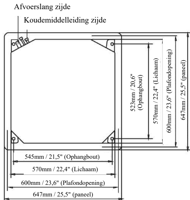
Compacte modellen afmetingen van het gat in het verlaagde plafond
