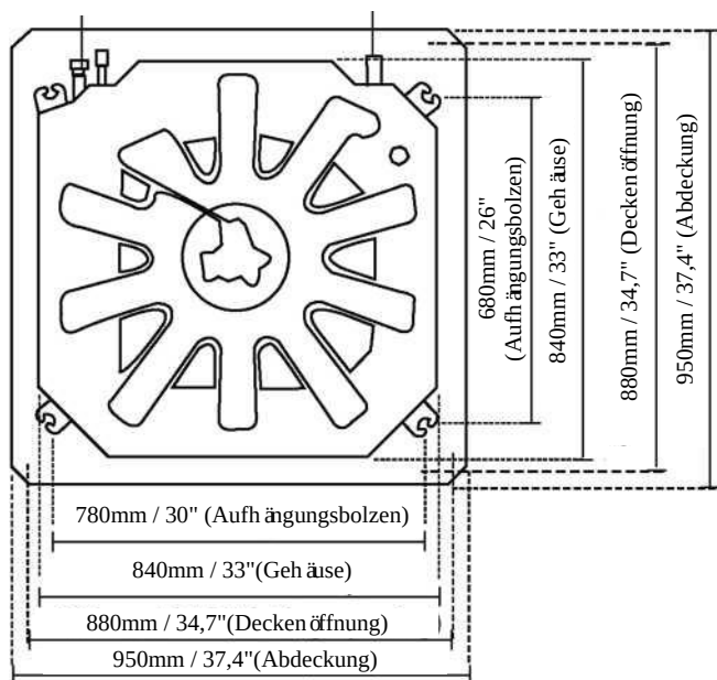
24-48K Klassische Modelle Abmessungen der Öffnung in der Zwischendecke
