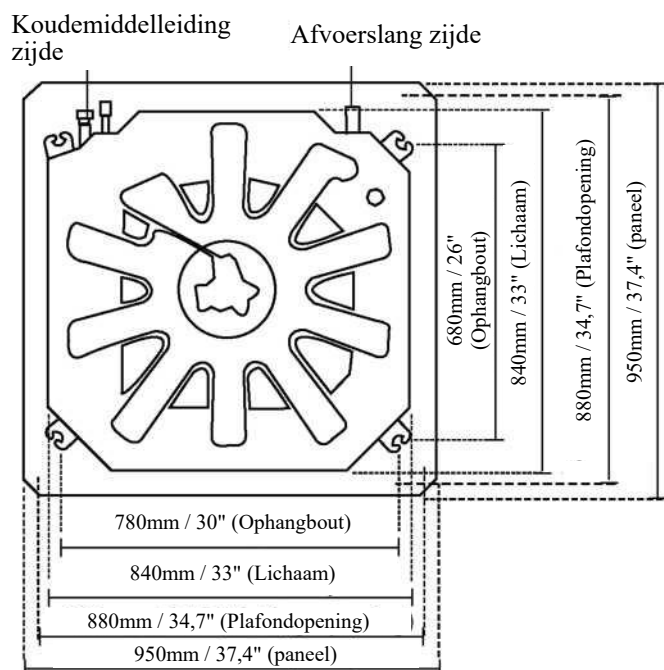
24-48K Klassieke Modellen afmetingen van het gat op het verlaagde plafond
