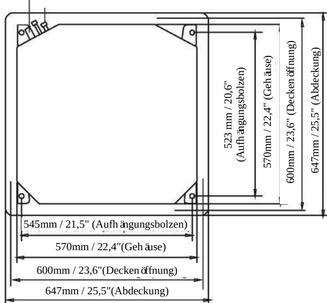
Kompakte Modelle Abmessungen der Öffnung in der Zwischendecke
