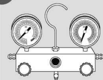
Évacuer le système de réfrigération
